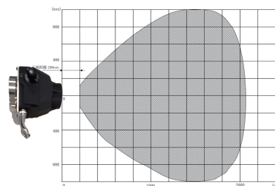
【旋回時電線検知センサー】
