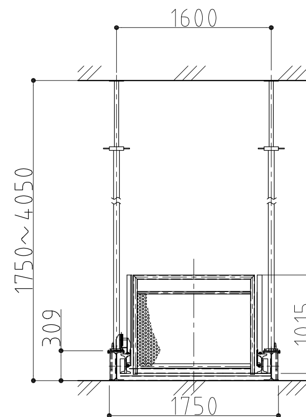
側面図
