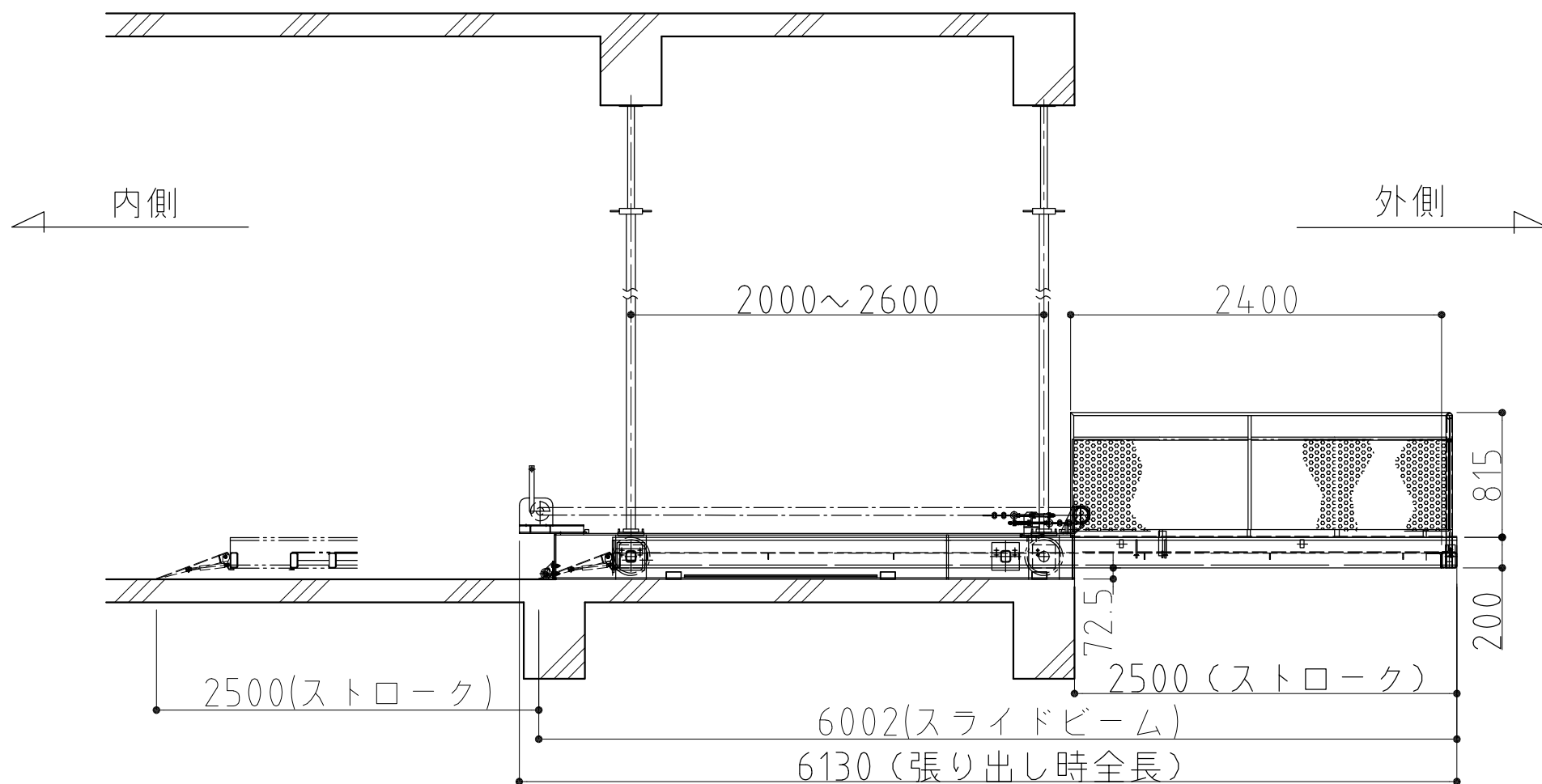
正面図
