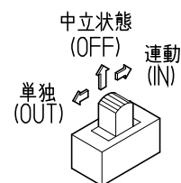
スライドスイッチ詳細図
