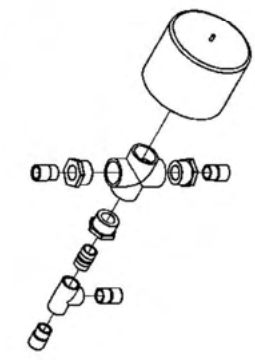
(吸込ロセット組立詳細図)
