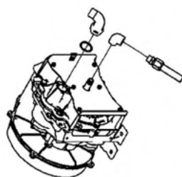
(コンプレッサ本体組立詳細図)
