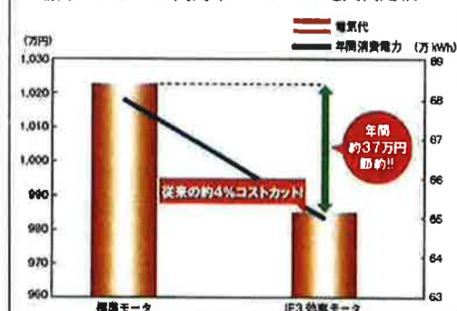
標準モーターと高効率モーターの電気代比較
