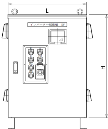
外形図
