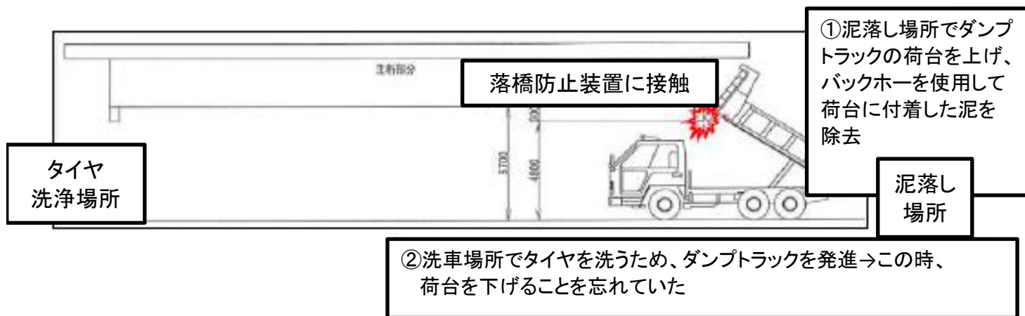
・落橋防止装置損傷状況
