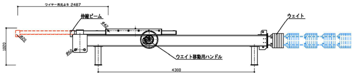
正面図
