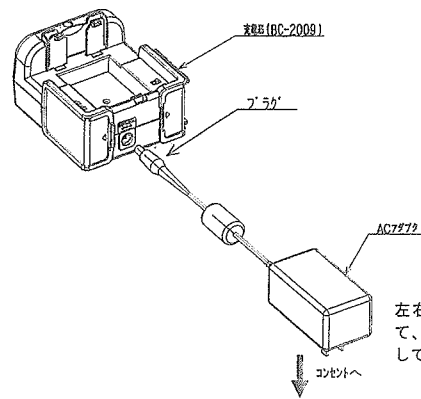
【充電器とACアダプタの接続】
