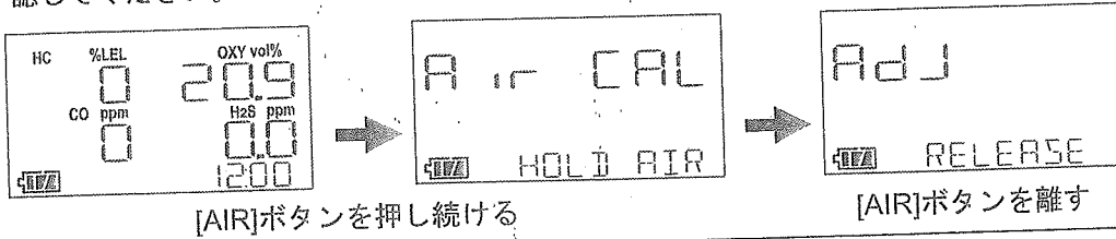
AIR ボタン
