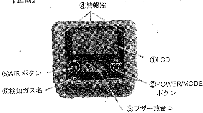
【正面】
