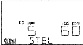
STEL 値表示(※1)
