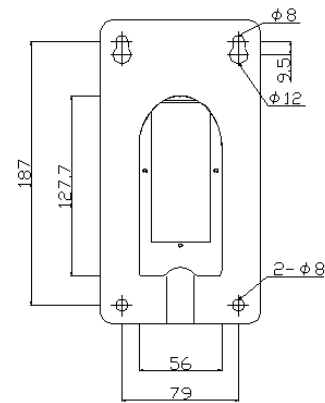
【壁付けブラケット壁面寸法】
