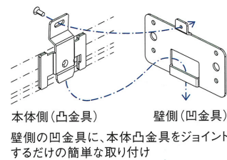
[取付金具]
