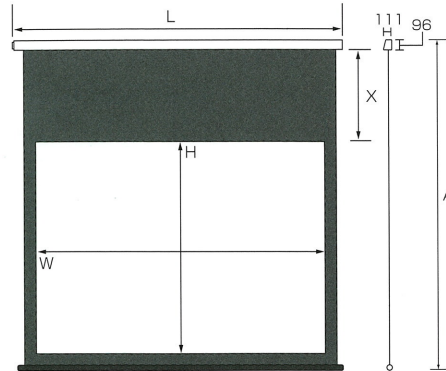
寸法図(単位:mm)
