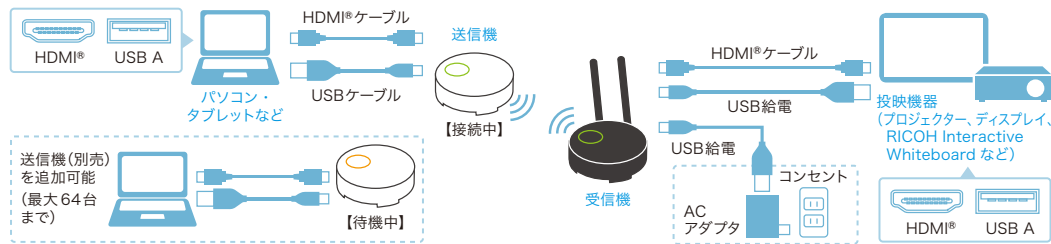
機器構成図
