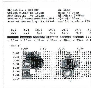
①グリッド機能を利用した測定結果のコンター図の印刷例
