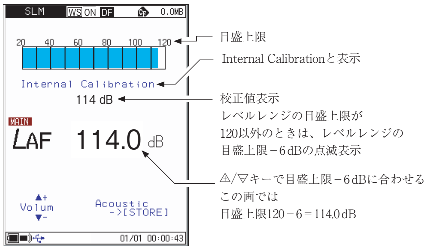
騒音計モード表示
