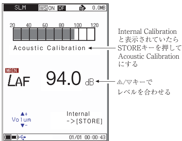
騒音計モード表示
