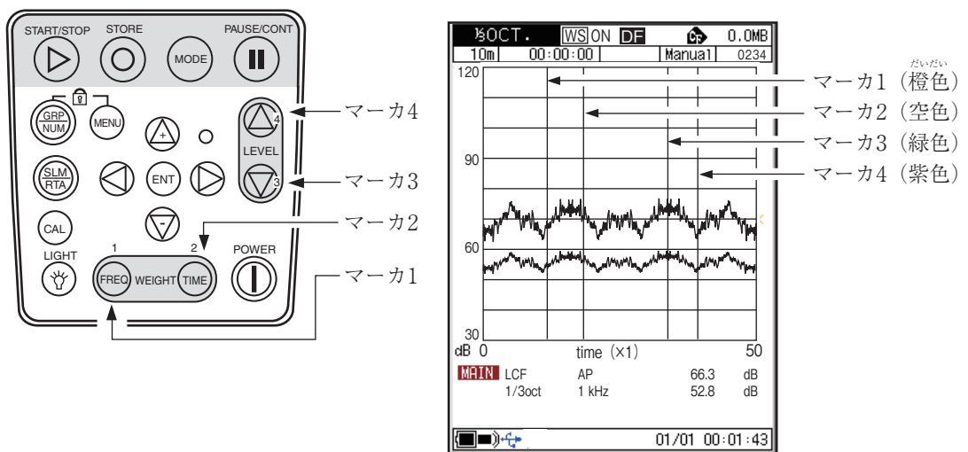
T-L表示画面
