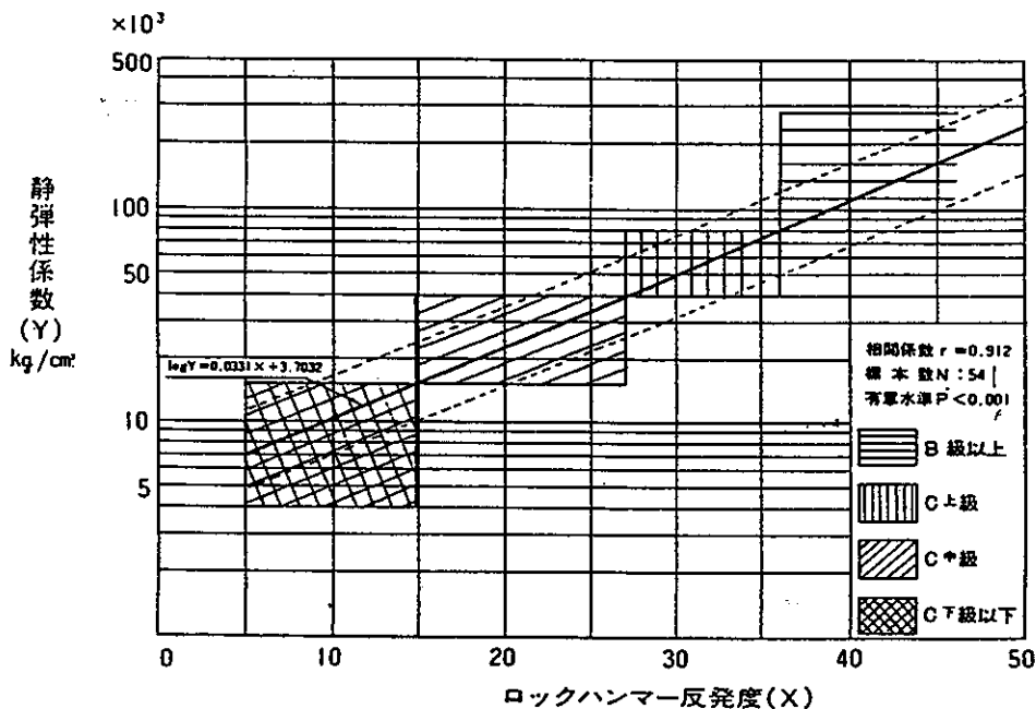
ロックハンマー反発度と { 岩盤等級 静弾性係数 } との関係
