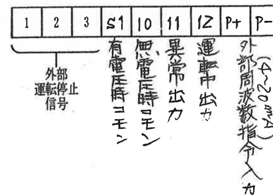
T B 2 (信号線端子台)
