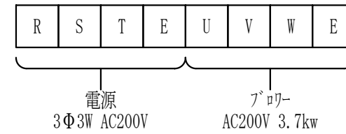
T B 1 (動力端子台)
