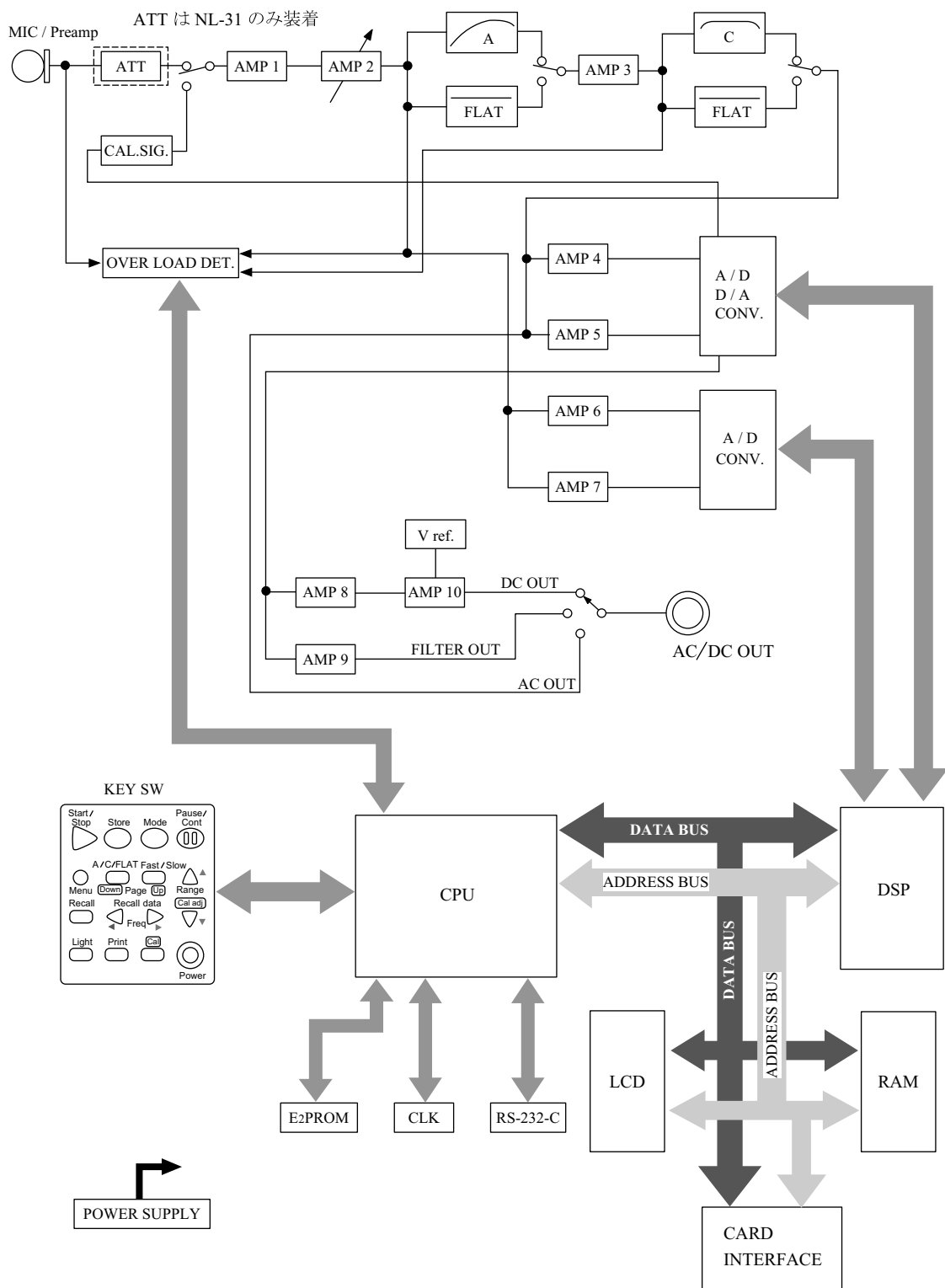
NL-21 / NL-31 ブロックダイヤグラム
