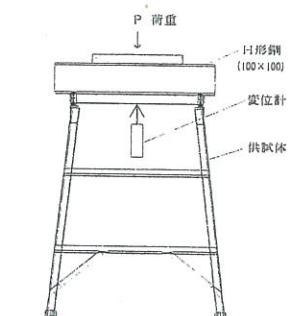
正面図
