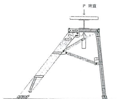
側面図
