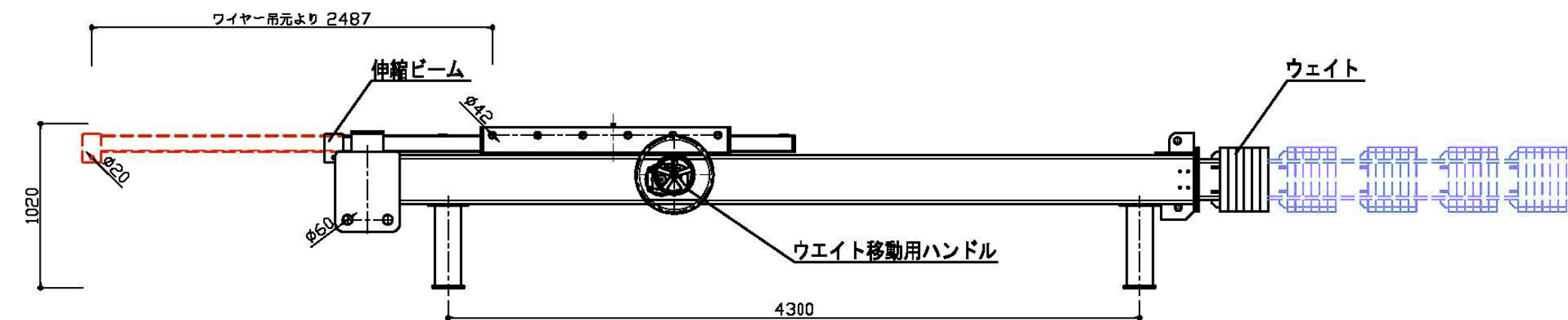
正 面 図
