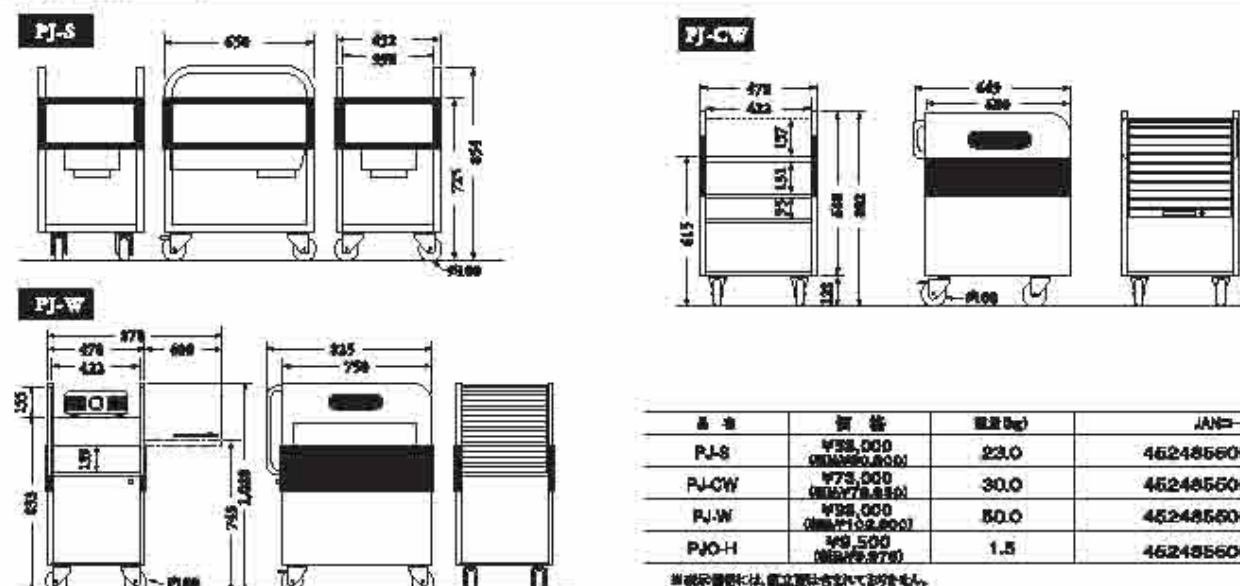
寸法図(単位:mm)
