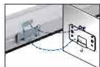
壁面への取り付け
