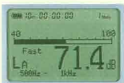
ユニバーサルフィルタカード NX-21VA (1/3オクターブバンドステップ)
