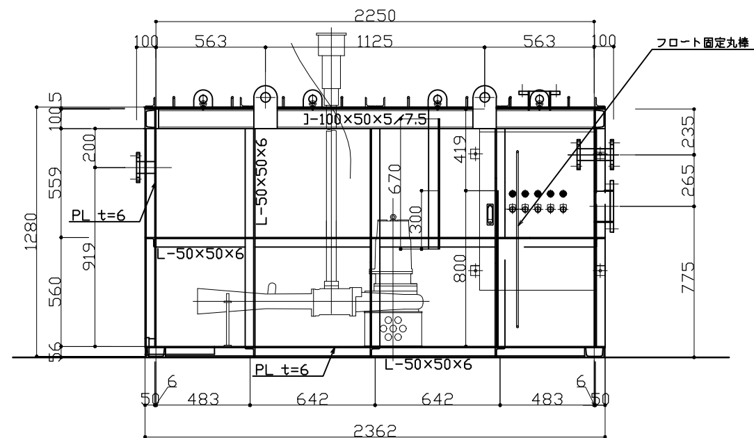
正面図
