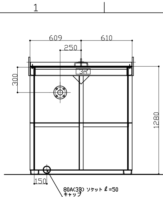
側面図
