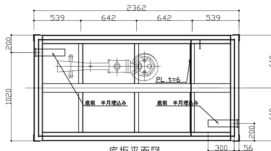
底板平面図
