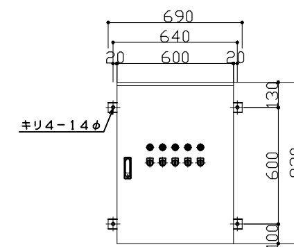
制御盤正面図
