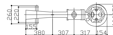
設置エジェクター: 22BER3
