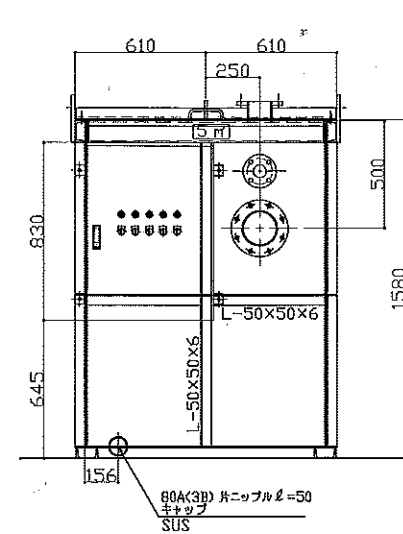
側面図
