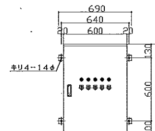
制御盤正面図
