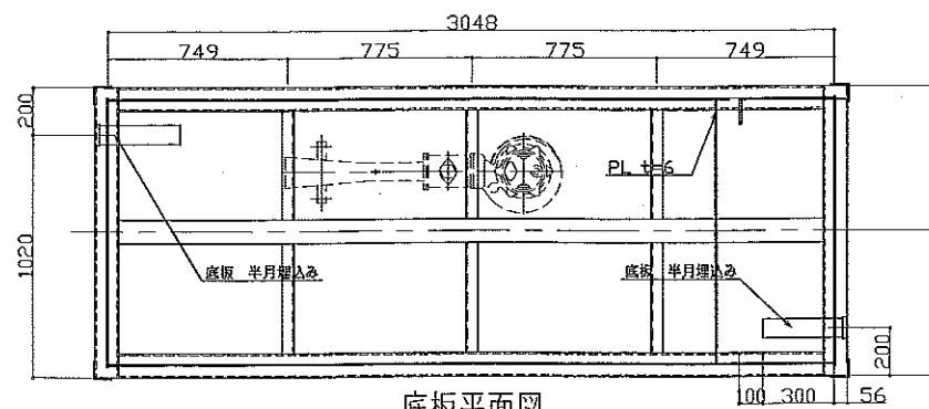
底板平面図
