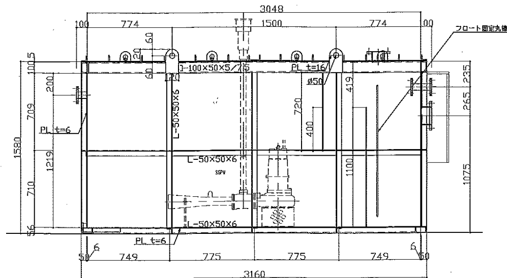
正面図
