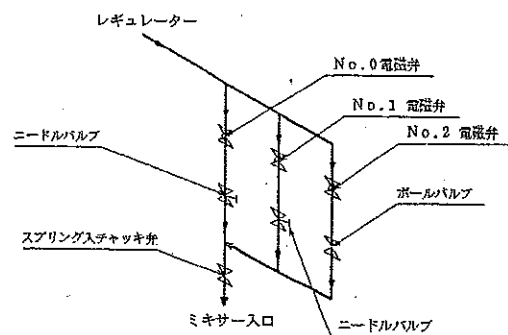
CO 2 ガス配置系統図
