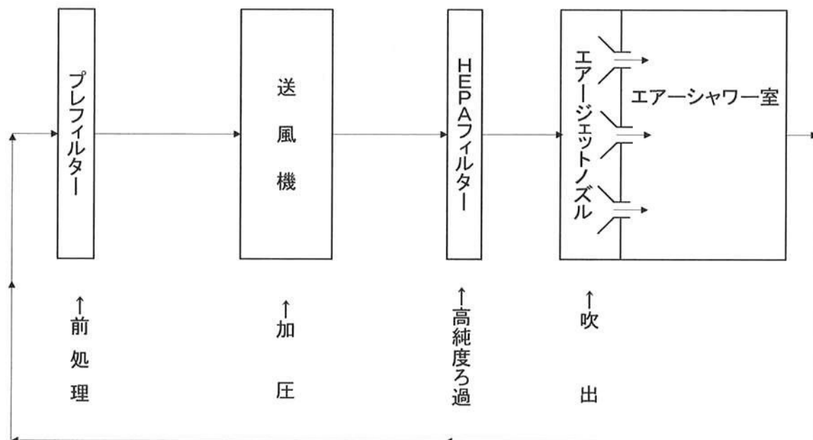
図一1 エアークンの浄化要素
