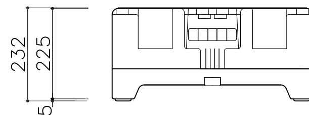
側面図（折りたたみ時）
