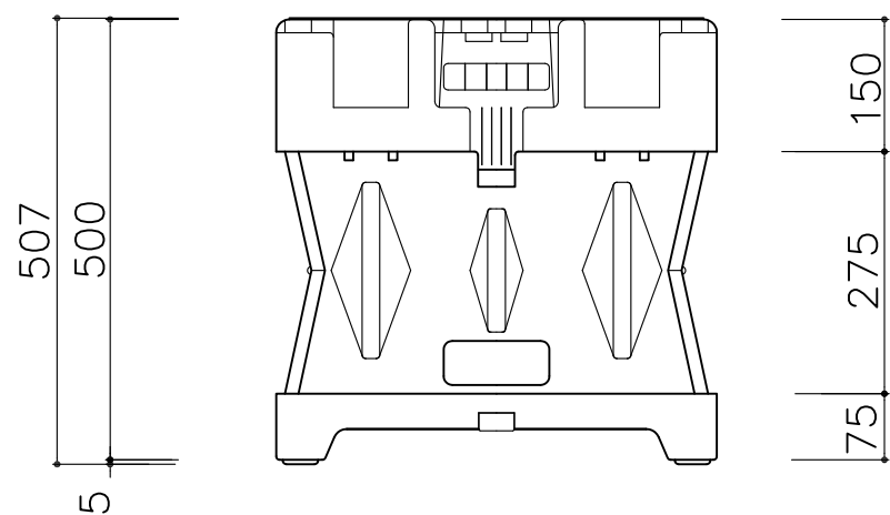
側面図（組立時）
