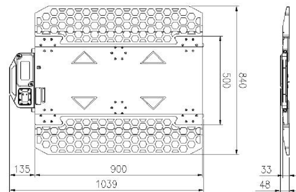
計量PAD寸法図
