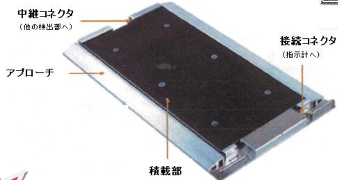
本体外観
